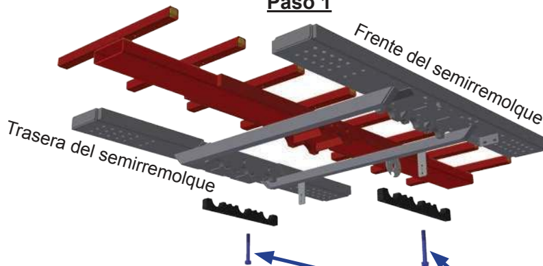
Tuerca de vástago estacionaria (sin ranuras) hacia la parte trasera del semirremolque
