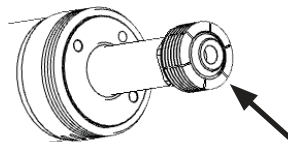
Tuerca de vástago ajustable (con ranuras) hacia la parte delantera del semirremolque
